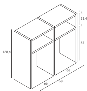
Struttura per lavatrice e asciugatrice, 2 ripiani
