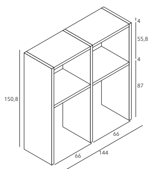
Struttura per lavatrice e asciugatrice, 2 ripiani
