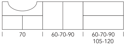
Basi lavabo sospese H.52 P.35/45/50
