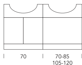
Basi lavabo a terra H.72 P.35
