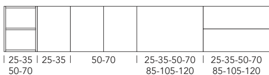
Basi contenitore sospese H.48 P.35/45/50
