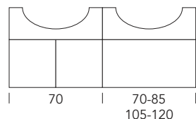
Basi lavabo sospese H.60 P.35
