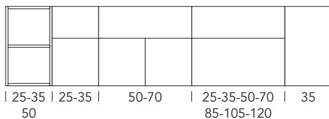
Basi contenitore sospese H.60 P.35/45/50
